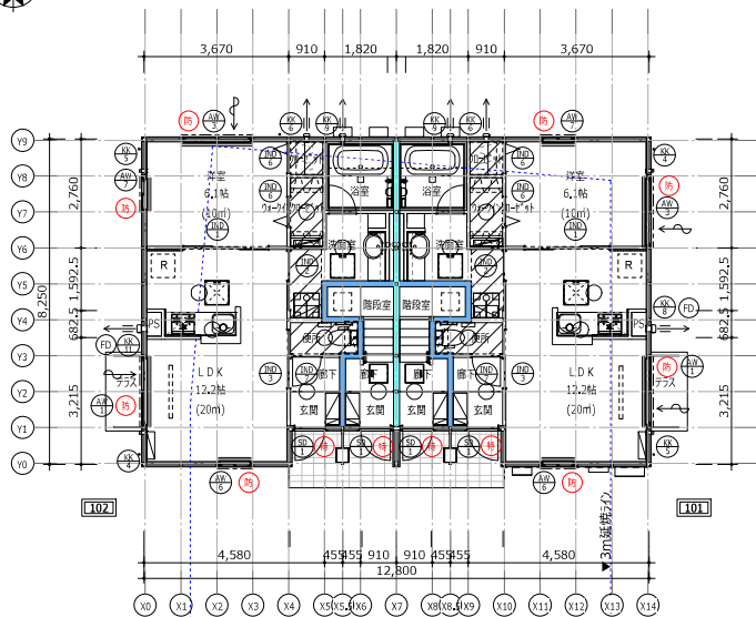
1階平面図 1/100
