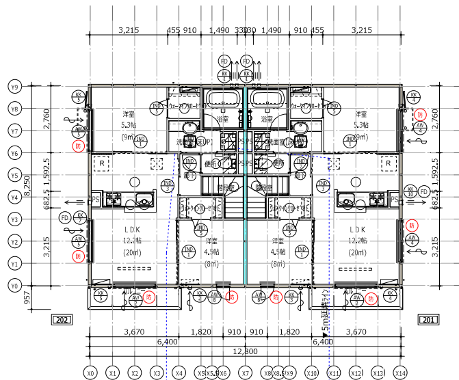
2階平面図 1/100
